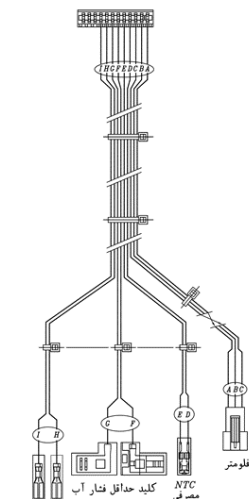
مازولیشن شیر گاز
